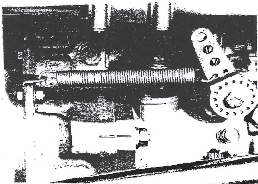
K2 Repères externes de calage vis à vis de la bride de pompe d'injection
