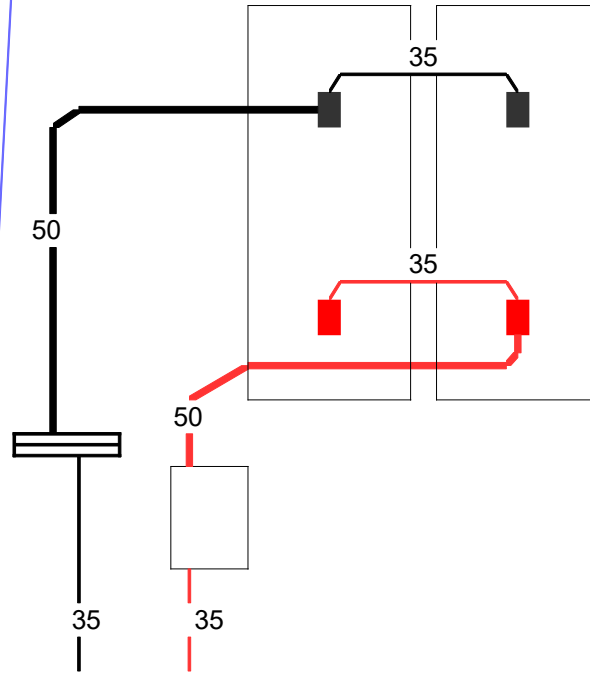
Nouveau montage (parallèle)
